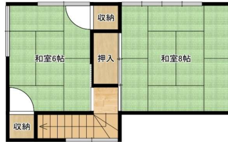
2階平面図
