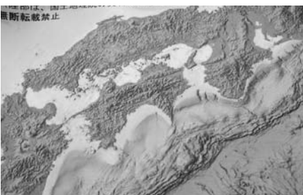
南海トラフ図（海上保安庁作製）
