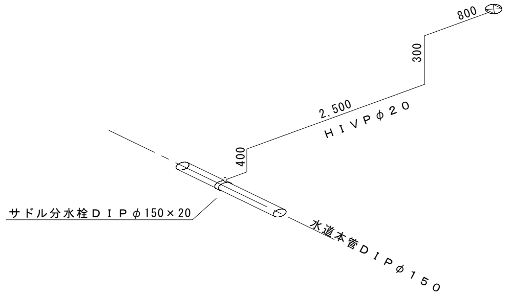
立体図
